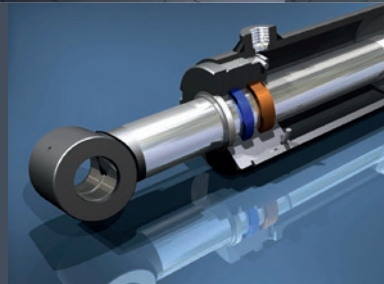
Hydraulikzylinder
