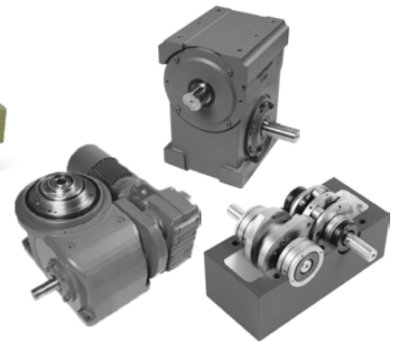
Rundschantische, kurvengesteuerte Schrittgetriebe und rollengetriebene Schrittschalengeräte von Ferguson
